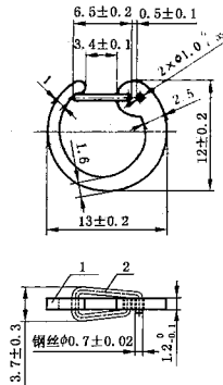
图1 弹簧卡扣结构和主要尺寸
